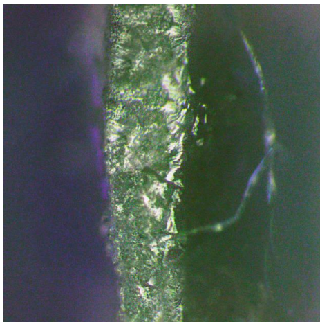
Разрез образца стопроцентно хлопчатобумажной ткани с нанесенным многофункциональным покрытием, увеличенный под микроскопом
